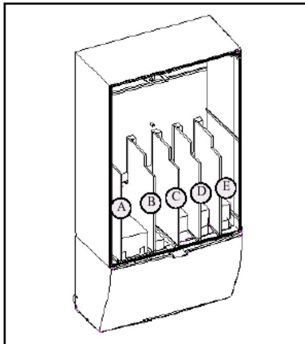
Rysunek 6-22. Sloty wraz z kartami WE/WY podstawowych i rozszerzających, znajdujące się na karcie sterującej.
