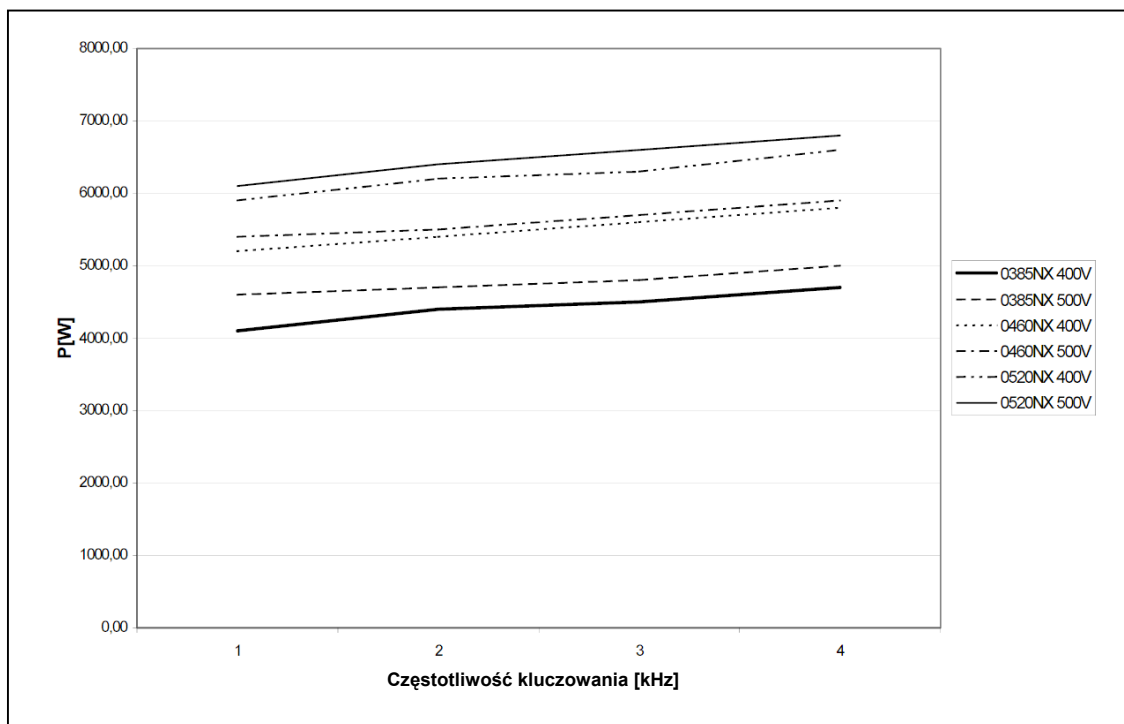
Rysunek 5-19. Straty mocy w funkcji częstotliwości klucowania; 0385...0520 NX_5.
