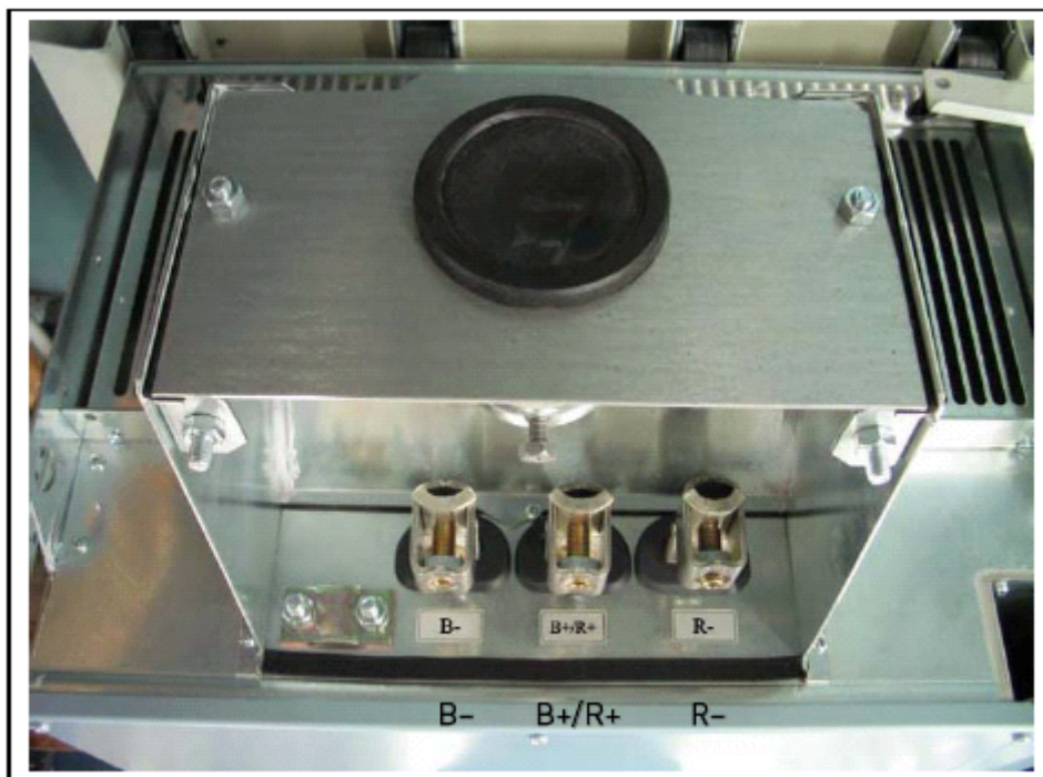
Rysunek 6-20. Zaciski DC i rezystora hamowania, podejście kabli od góry, wielkość mechaniczna FR9; zaciski obwodu DC oznaczone jako B- i B+, zaciski rezystora hamowania oznaczone jako R+ i R-.
