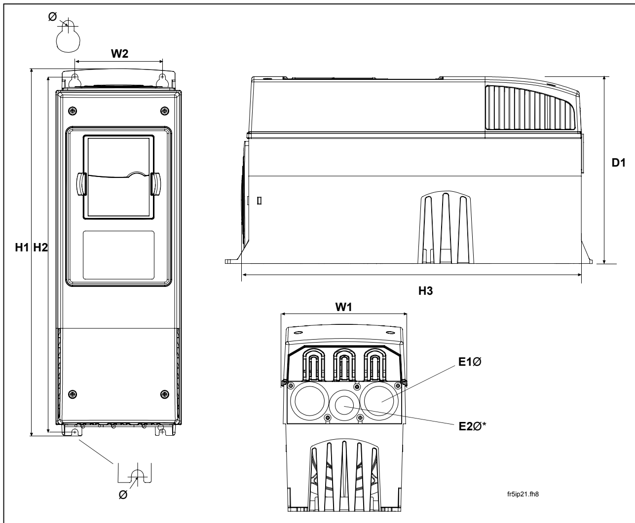
Rysunek 5.1. Wymiary montażowe.
