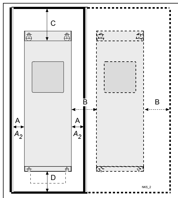
Rysunek 5-11. Przestrzeń montażowa.
