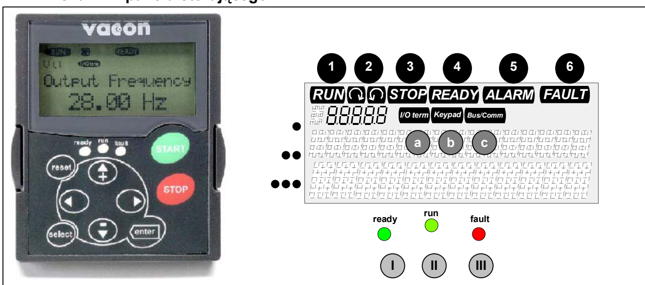
Rysunek 7-1 Panel sterujący Vacon NX wraz ze wskaźnikami stanu pracy napędu.
