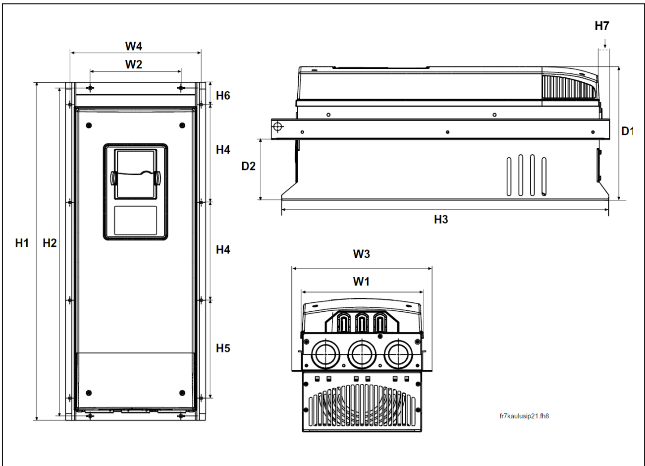
Rysunek 5-4. Wymiary montażowe, montaż kołnierzowy. Wielkość mechaniczna FR7 do FR8.
