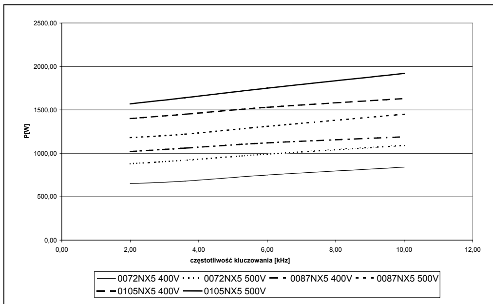
Rysunek 5-16. Straty mocy w funkcji częstotliwości kluczenia; 0072...0105 NX_5.
