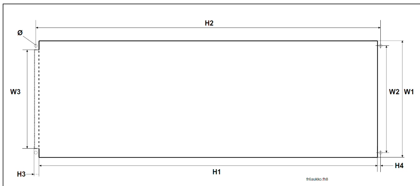
Rysunek 5-3. Wymiary otworu do montażu kołnierowego. Wielkość mechaniczna FR4 do FR6.
