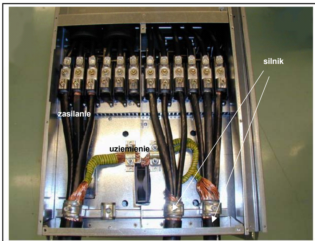
Rysunek 6-19. Podłączenie kabli w Vacon NX, wielkość mechaniczna FR9.
