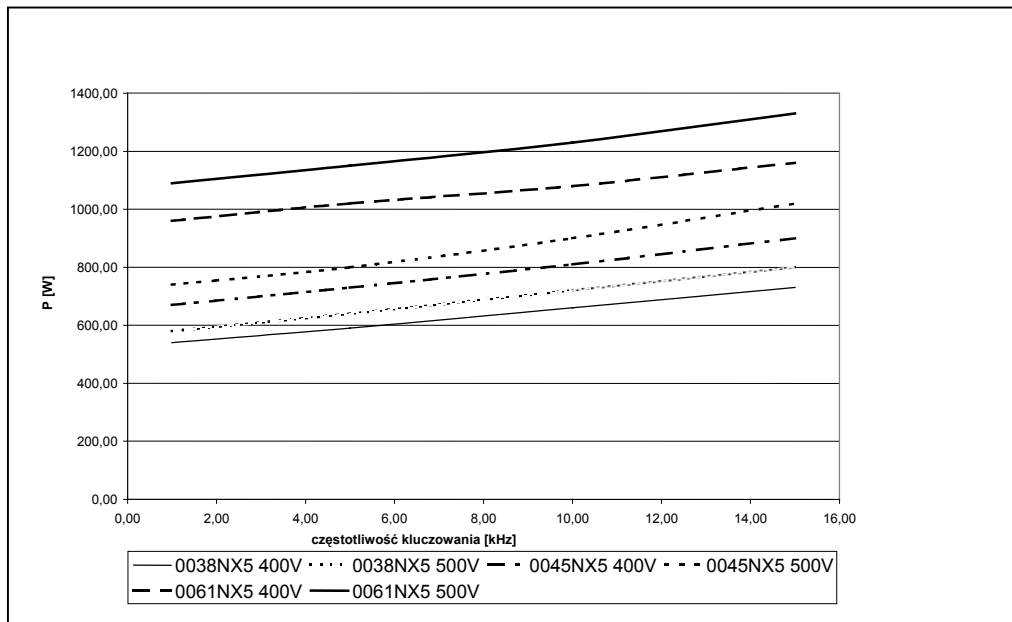
Rysunek 5-15. Straty mocy w funkcji częstotliwości kluczenia; 0038...0061 NX_5.
