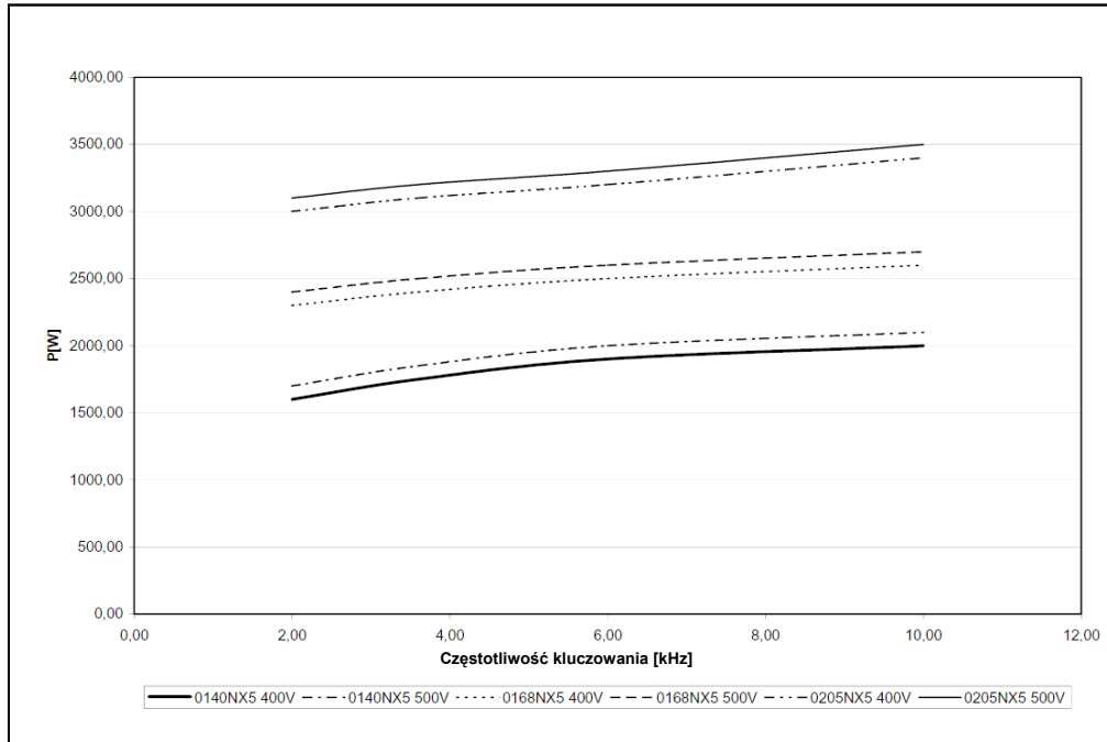
Rysunek 5-17. Straty mocy w funkcji częstotliwości klucowania; 00140...0205 NX_5.
